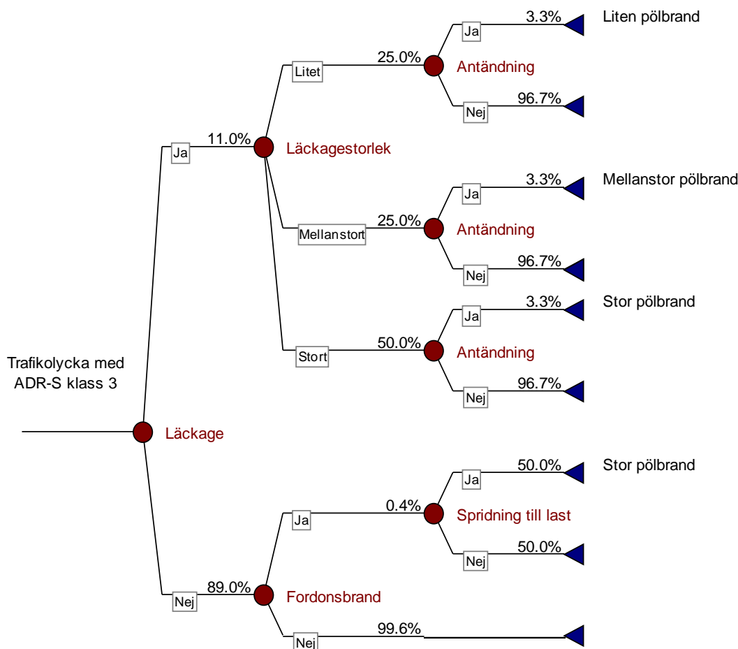
Figur 10. Händelsetråd med sannolikheter för ADR-S klass 3. Sannolikhet för läckage regleras av index, se Tabell 4
