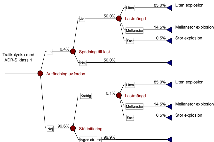
Figur 7. Händelsetråd med sannolikheter för ADR-S klass 1.
