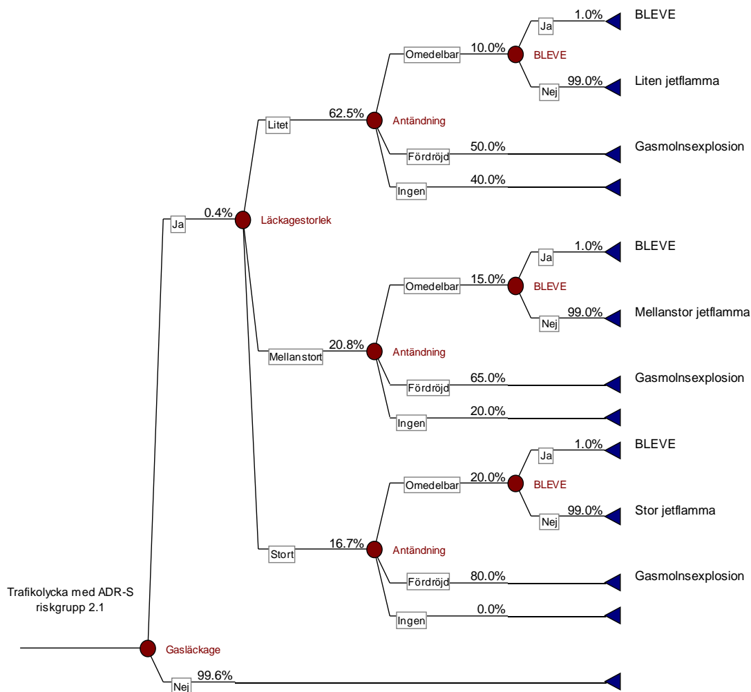
Figur 8. Händelseträäd med sannolikheter för ADR-S klass 2.1.
