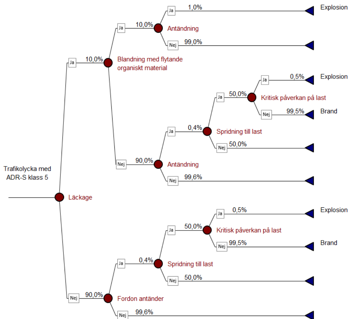
Figur 11. Händelsetråd med sannolikheter för ADR-S klass 5.
