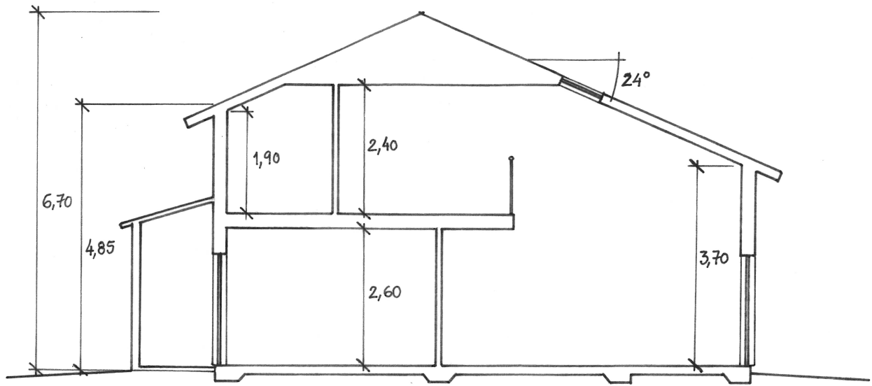
SEKTION A-A
